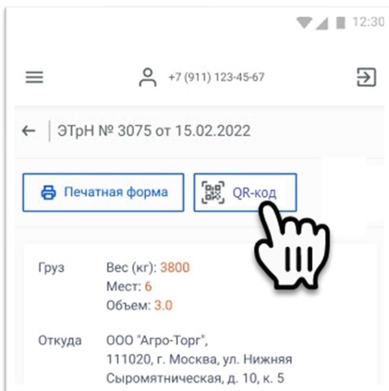
Рисунок 16. Кнопка «QR-код»
