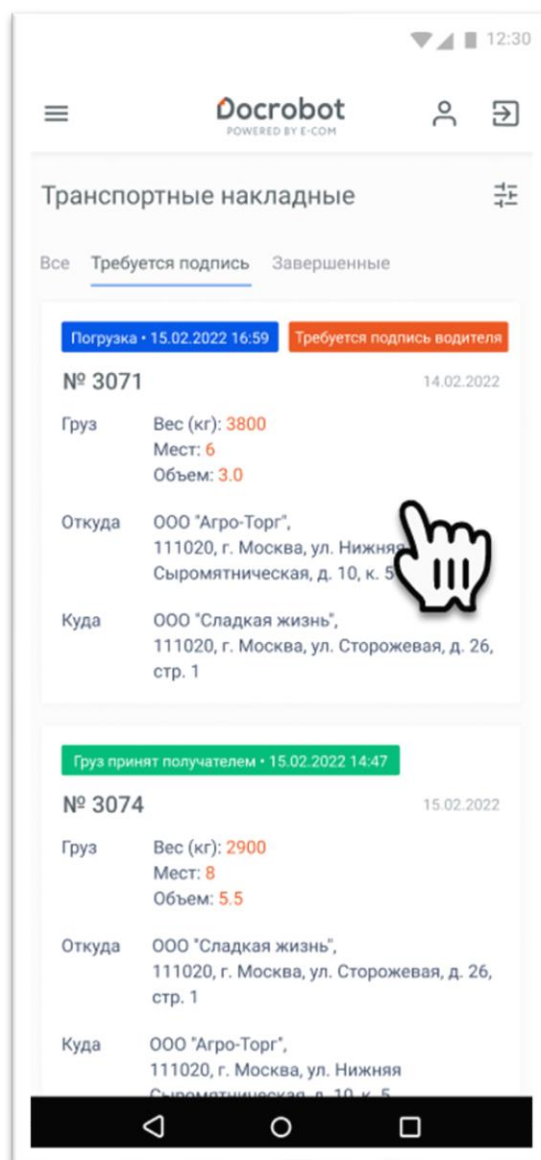
Рисунок 9. Открытие накладной
