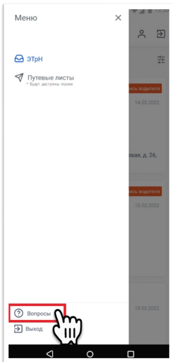
Рисунок 19. Вкладка «Вопросы»
