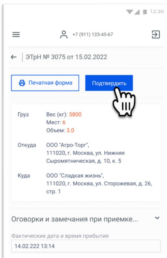
Рисунок 14. Подписание накладной
